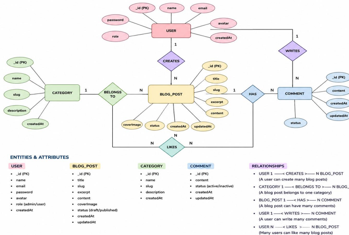
BlogNest – ER Diagram
